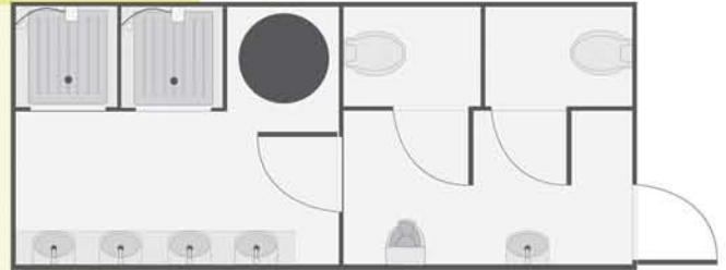
Kontener Sanitarny Standard
