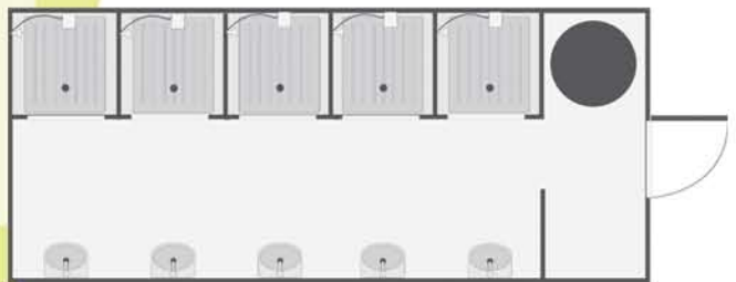
Kontener Prysznicowy z przedsionkiem
